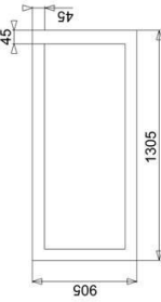
SUPERFICIE APPOGGIO A PAVIMENTO FLOOR SUPPORT AREA
