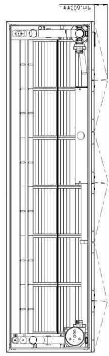
LATO ISPEZIONE INSPECTION SIDE
