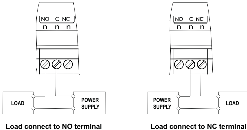
Fig. 9. Digital/Relay Outputs
